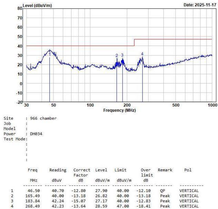
图 6-6 辐射测试水平方向
