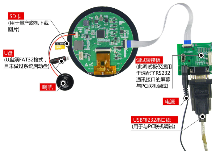
图 1-3 调试工具图
