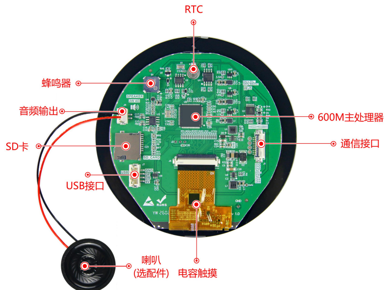
图 1-2 硬件配置图
