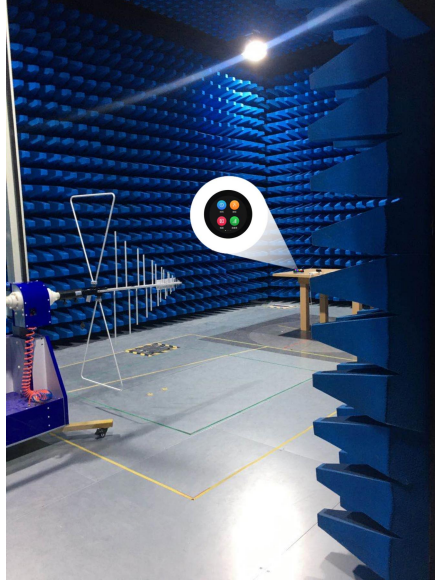
图 6-5 辐射测试图
