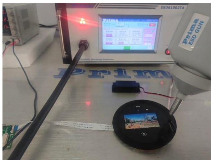
图 6-2 ESD 测试图
